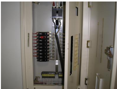
配電盤からの電源確保の例
